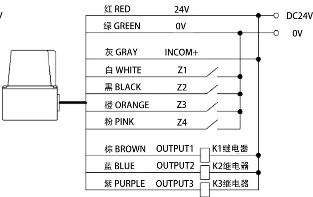
NPN输出形式接线图
