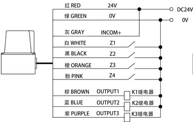
PNP输出形式接线图
